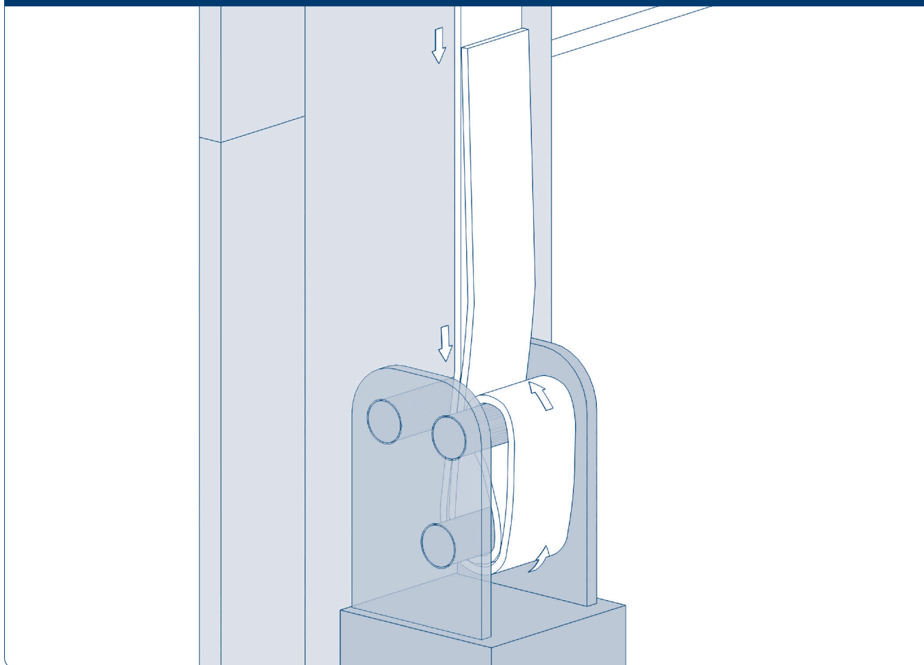
Рис. 6.3.3. Заправка ремня в противовес
