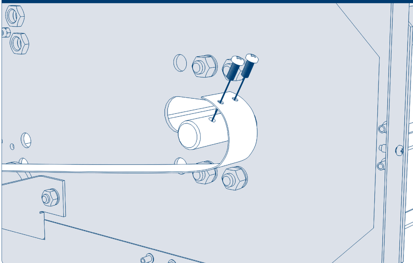
Рис. 6.3.1. Крепление ремня к валу
